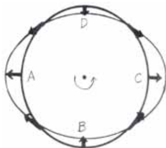
Fig3 :起潮力により変形を受け、回転楕円形となる平衡海面。
