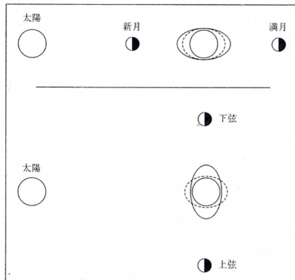
Fig4 :大潮(上段)と小潮(下段)の時の月の起潮力による平衡海面(実線)と太陽の起潮力による平衡海面(破線)
