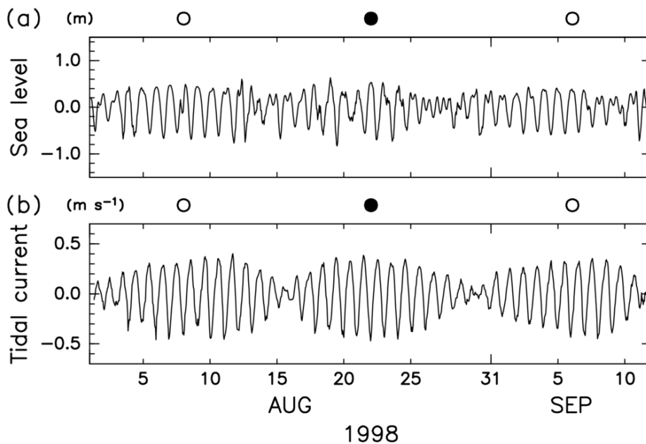
Fig 1 : サハリン島東岸沖の(a)潮位と(b)潮流の南北成分。 ●は満月、○は新月。 Ono et al.(2008)より加筆。
