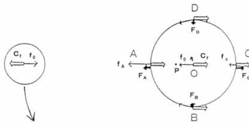
Fig 2 : 引力( f_0 \cdot f_A \cdot f_C )と遠心力( C_f : 白矢印)と起潮力( F_A \cdot F_B \cdot F_C \cdot F_D )。Oは地球の中心、Pは地球と月の共通重心を表す。Pは地球の内部に位置する。
