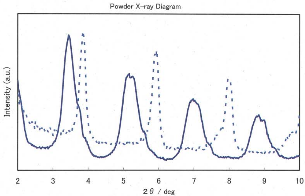
図1. n-hexatriacontane の粉末X線回折図形
